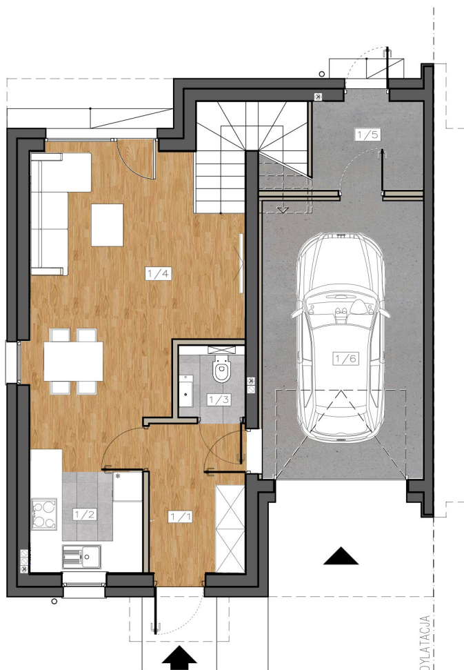
RZUT PARTERU
